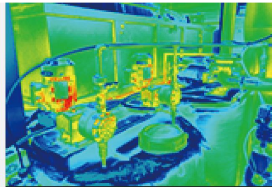
工場内のサーマルカメラ撮影した様子
